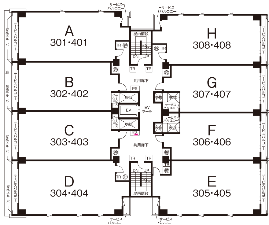
■ 3・4階平面図
