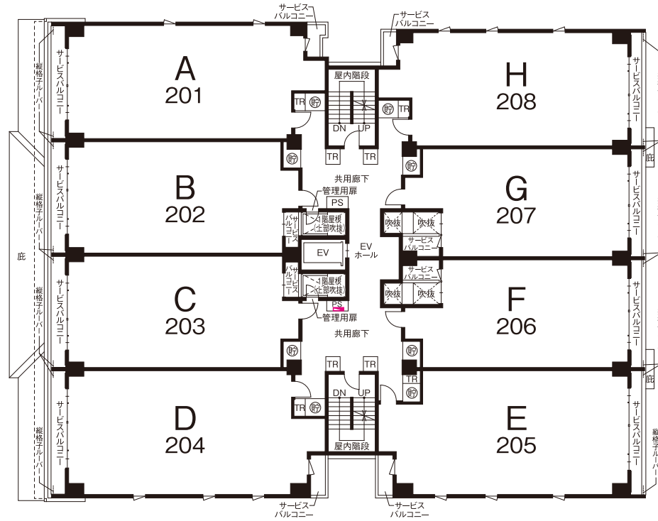
■ 2階平面図
